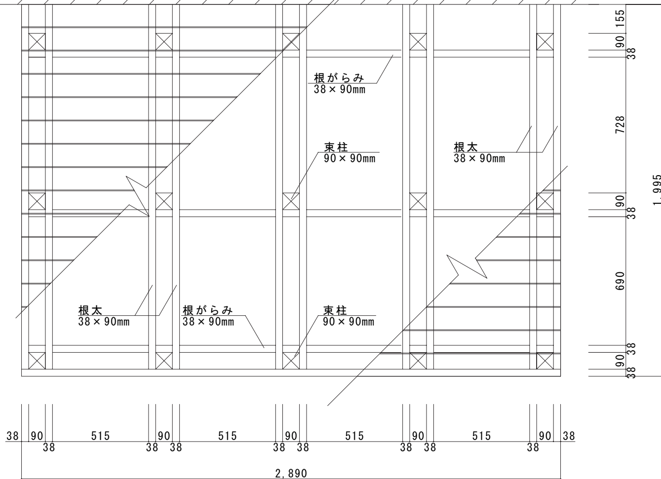
平 面 図
