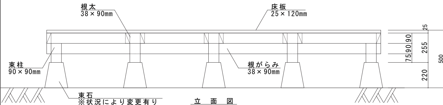
立 面 図
