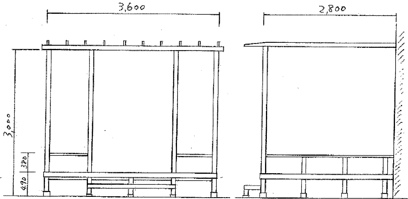
立面図 S = 1 : 50
