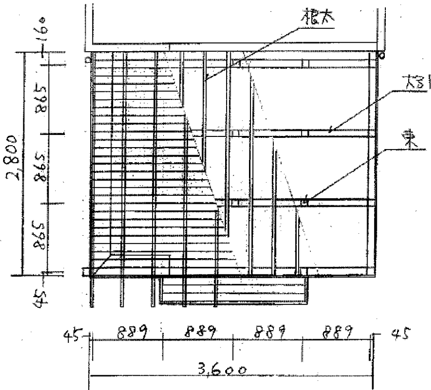
平面図 S = 1 : 50
